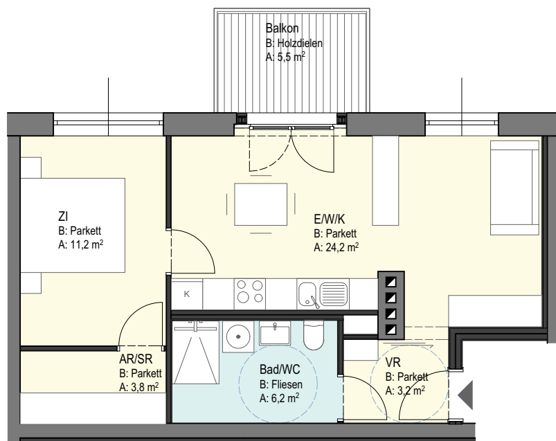
Grundriss 1:100
