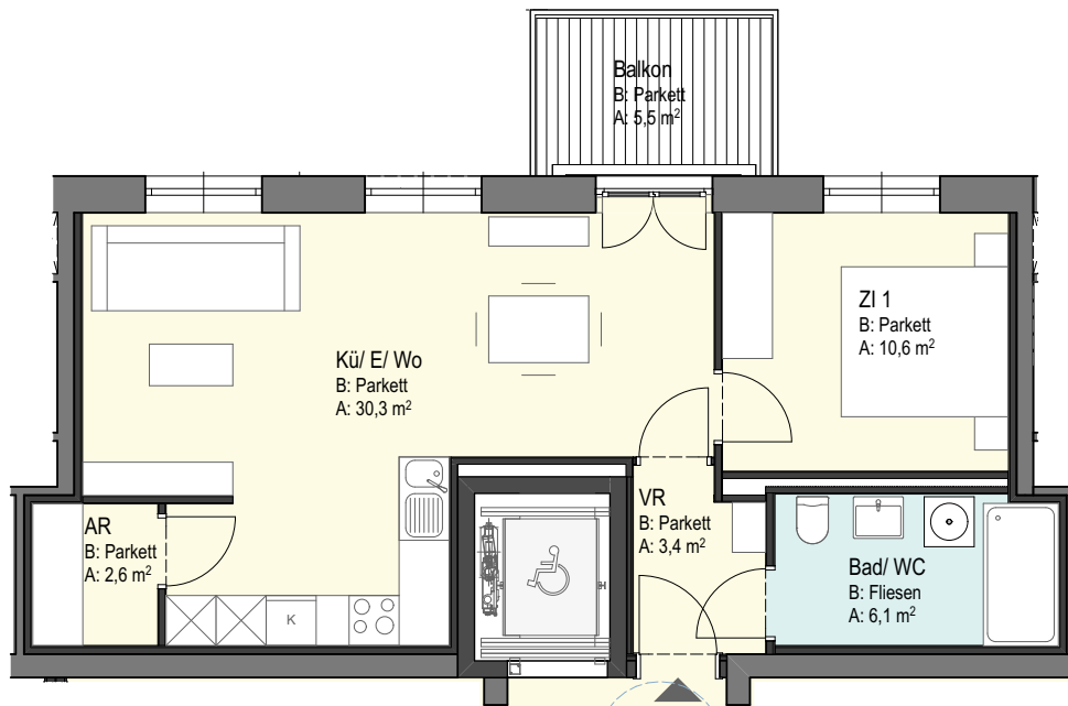
Grundriss 1:100
