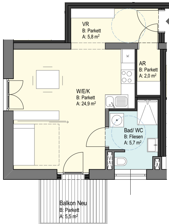
Grundriss 1:100
