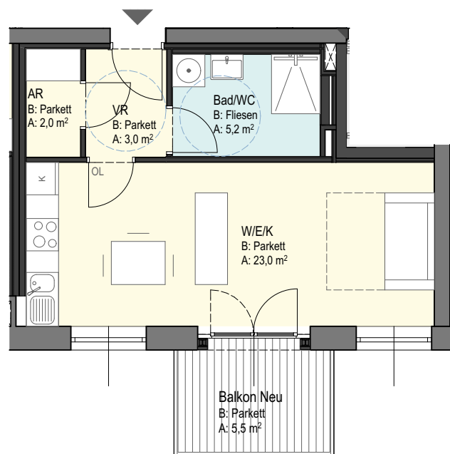
Grundriss 1:100
