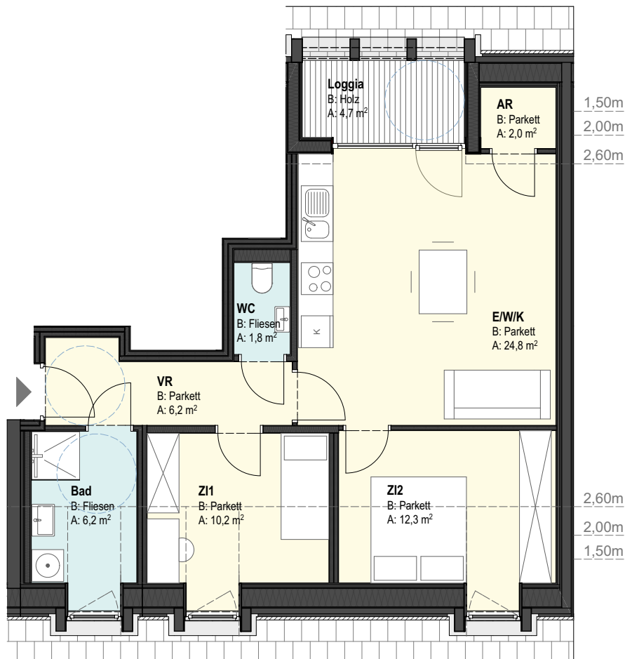
Grundriss 1:100
