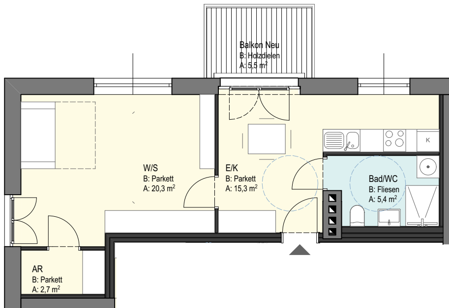
Grundriss 1:100
